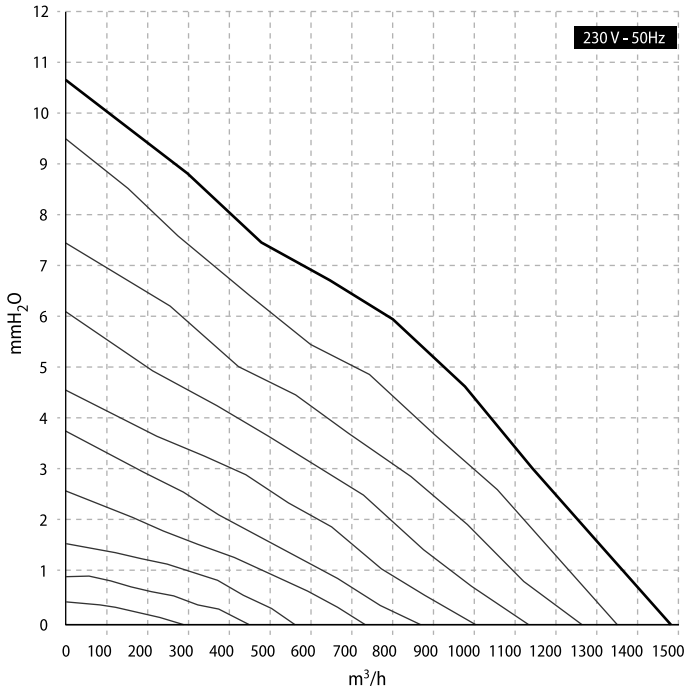
CAUDAL PRESIÓN FCET
