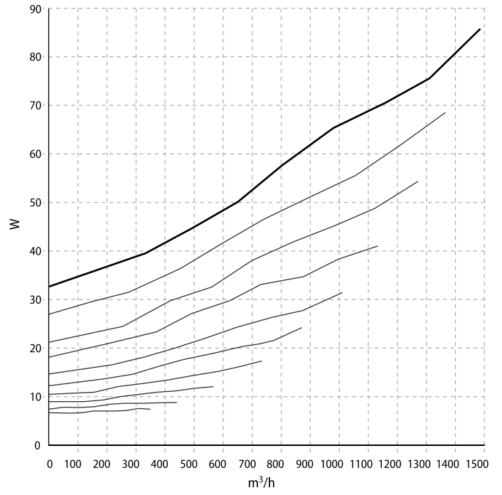
POTENCIA ABSORBIDA FCET
